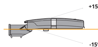
Horizontale Montage
