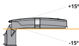
Vertikale Montage
