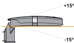
Montaggio verticale
