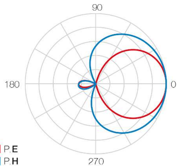
Diagrama de radiação
