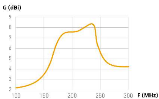
Frekvenssvar
