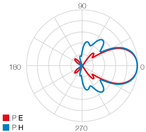
Diagrama de radiación
