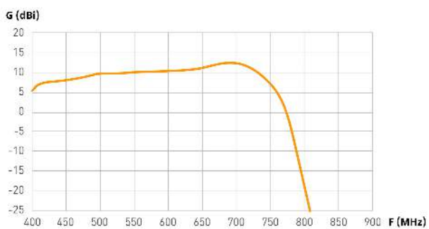
Diagrama de radiación
