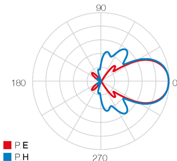
Charakterystyka promieniowania
