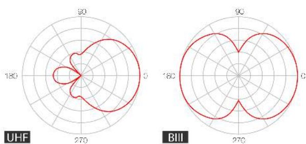
Charakterystyka promieniowania
