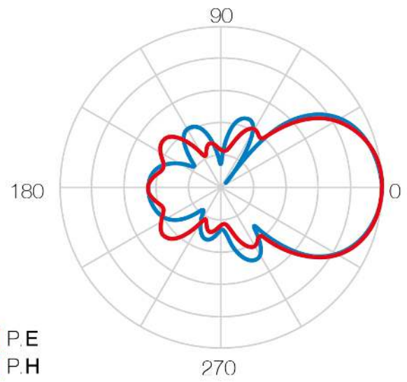
Strålningsmönster
