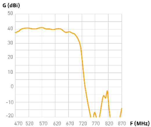
Charakterystyka promieniowania
