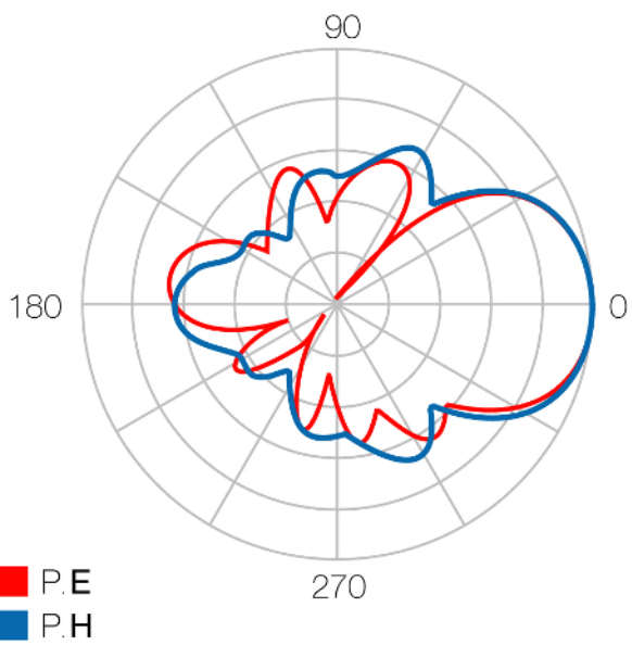
Charakterystyka promieniowania
