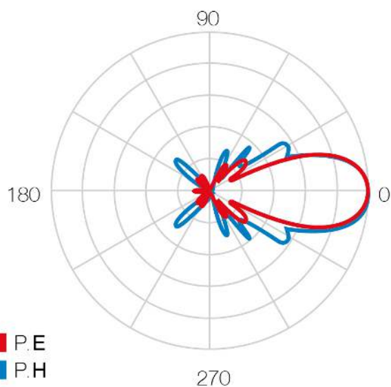
Diagrama de radiación
