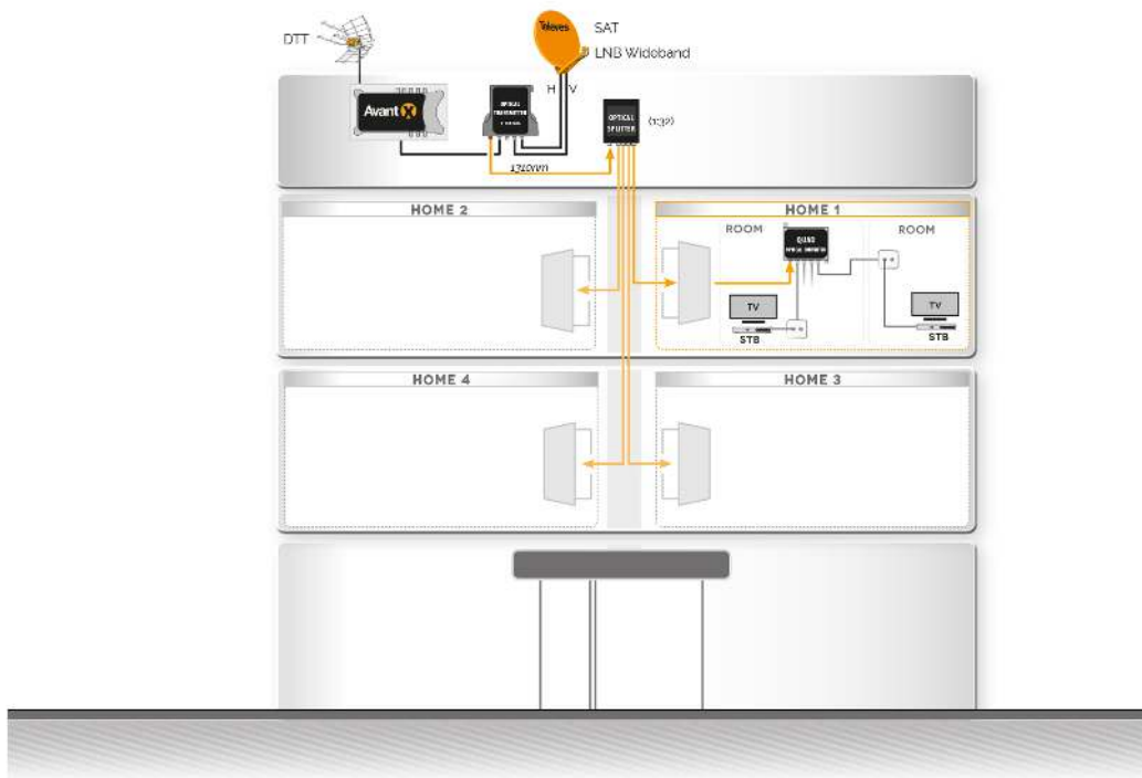
FTTR: Studentenwohnheim (DVB-T2 + SAT)
