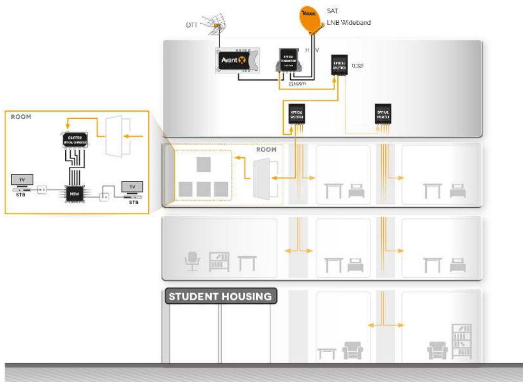
FTTB: Hotel (DVB-T2 + 3SAT)
