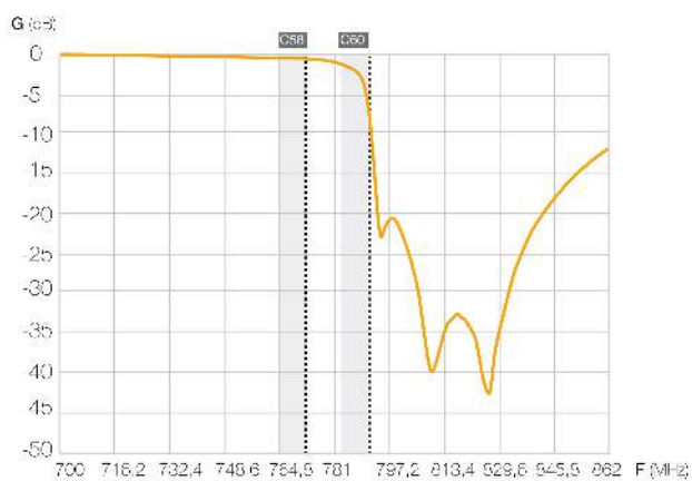
Frekvenssvar
