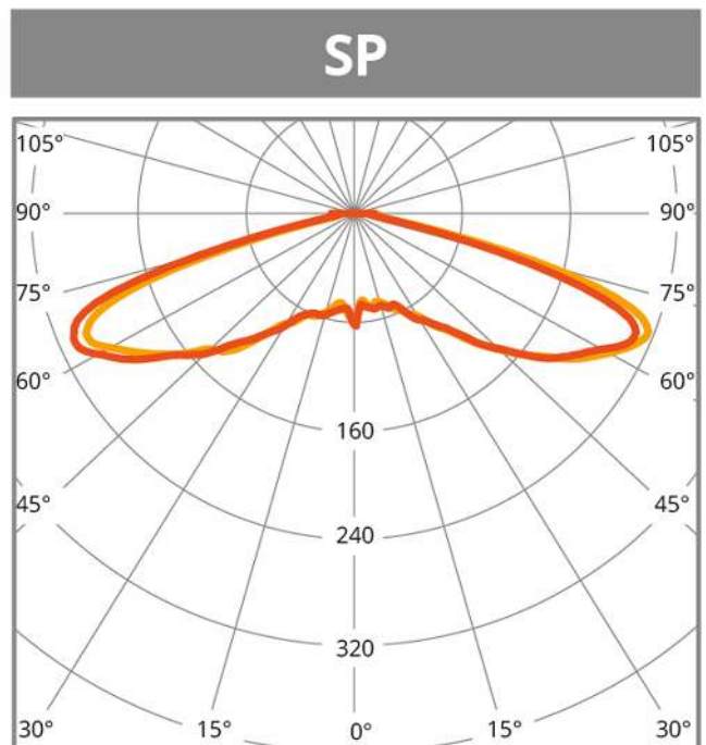
cd/klm ■ C0 - C180 ■ C90 - C270 \eta = 96\% Distribuzione luminosa
