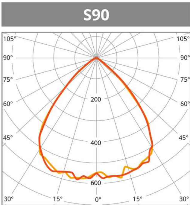
cd/klm ■ C0 - C180 ■ C90 - C270 \eta = 100\% Distribuzione luminosa
