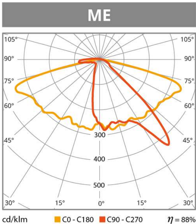
Distribución lumínica
