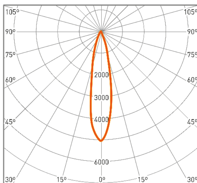
Distribución lumínica
