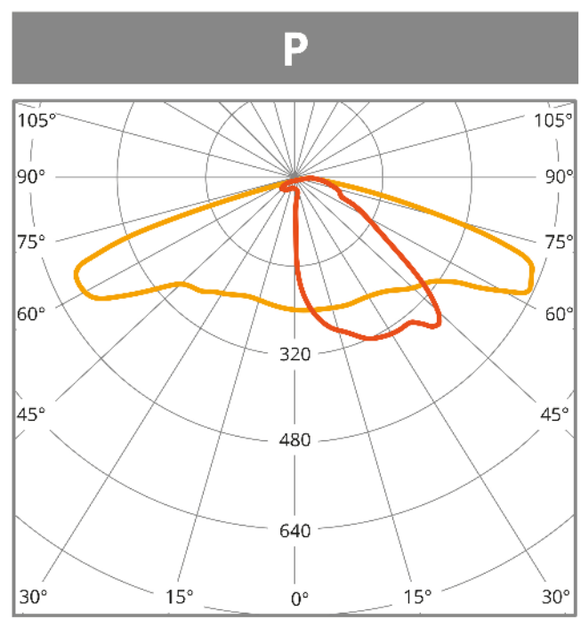
cd/klm ■ C0 - C180 ■ C90 - C270 \eta = 94\% Lichtverteilung
