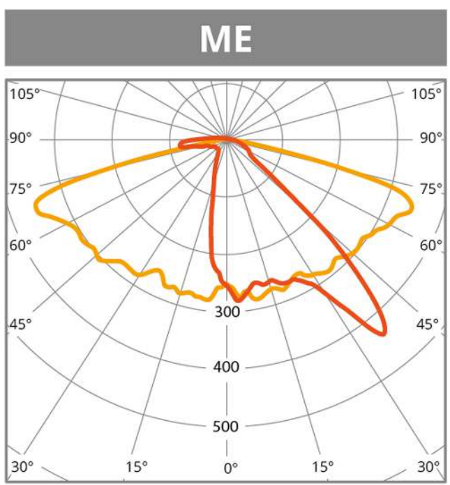
cd/klm ■ C0 - C180 ■ C90 - C270 \eta = 88\% Lichtverteilung
